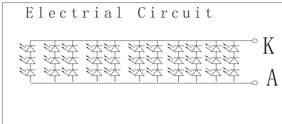
3串9并 27灯
